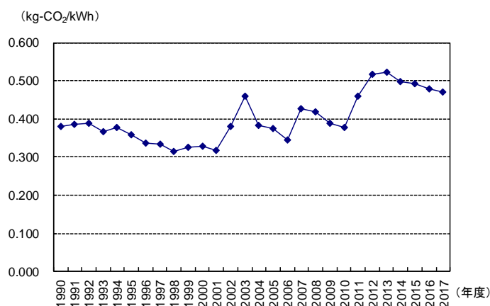
図 III-3 電力の二酸化炭素排出係数の推移
