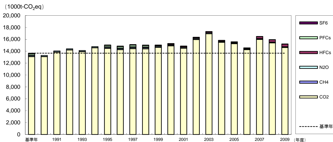
図 III-1 多摩地域の温室効果ガス排出量の推移
