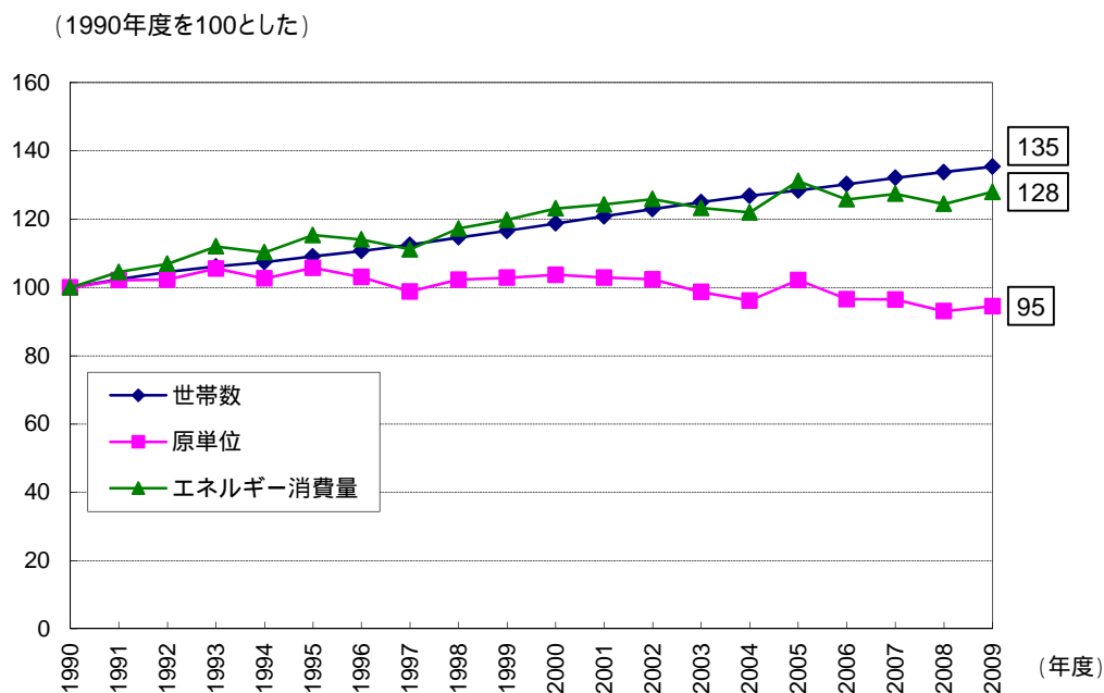
図 III-4 世帯数とエネルギー消費量
