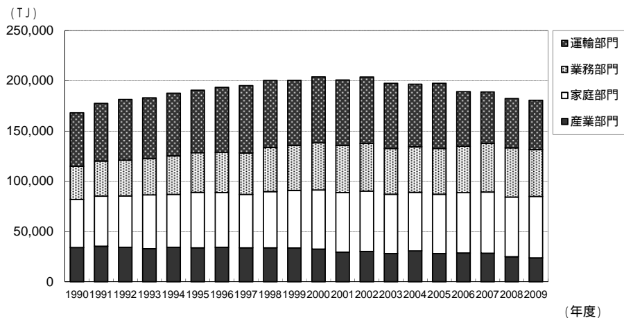
図 III-2 多摩地域のエネルギー消費量の推移
