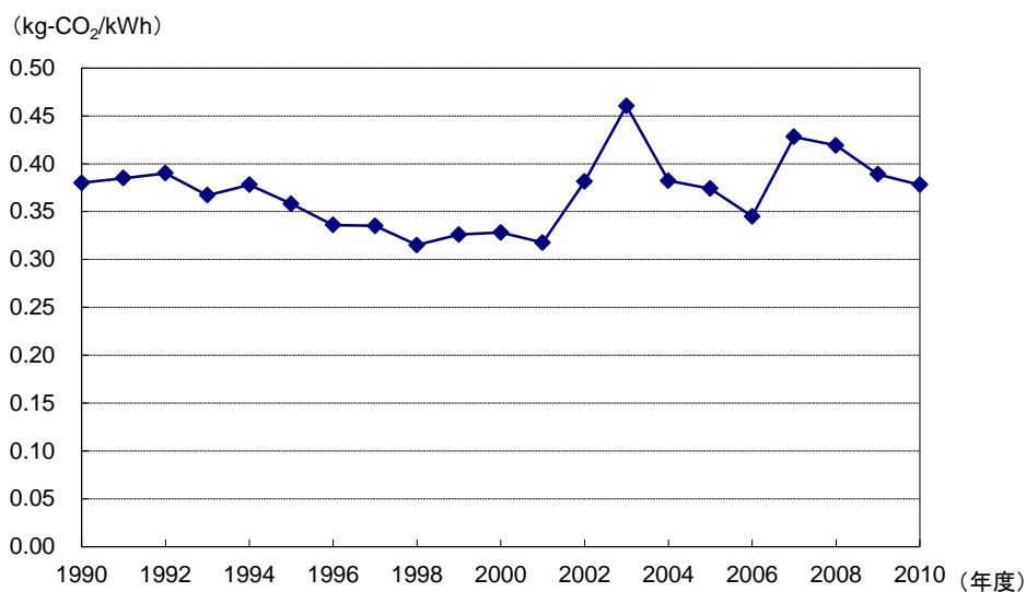
図 III-3 電力の二酸化炭素排出係数の推移
