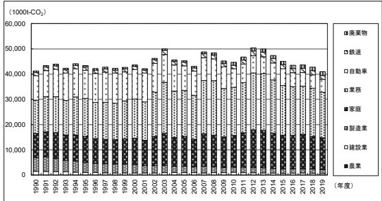
図 I-1 23 区における部門別二酸化炭素排出量の推移 (注) 二酸化炭素は温室効果ガス排出量の中で大半を占めるため、二酸化炭素排出量についての推移を掲載している。
