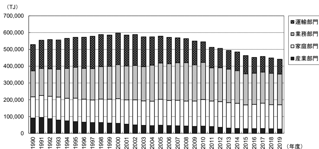
図 II-2 23 区のエネルギー消費量の推移
