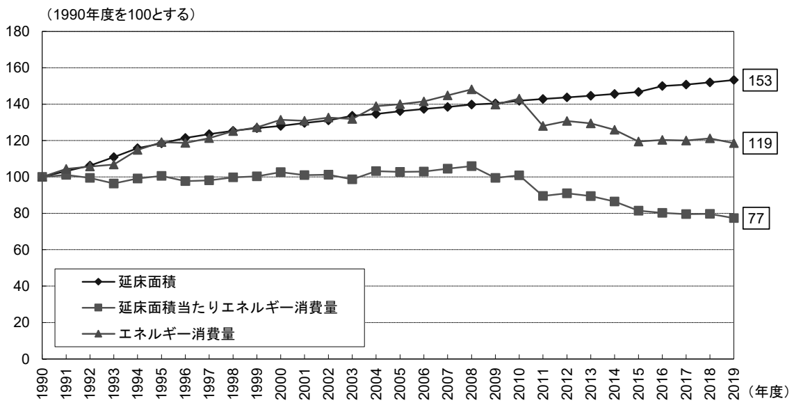
図 II-6 延床面積とエネルギー消費量
