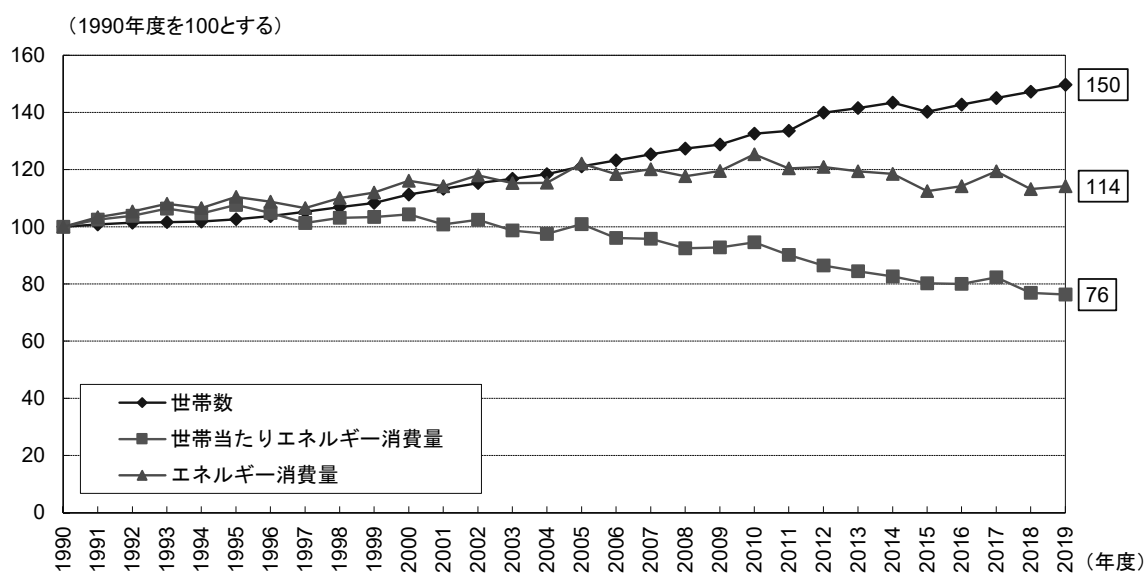
図 II-5 世帯数とエネルギー消費量
