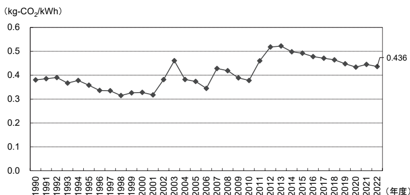
図 III-3 電力の二酸化炭素排出係数の推移
